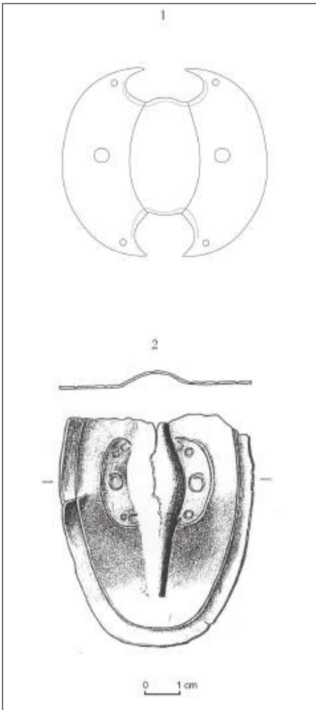
Fig. 7 1, Ricostruzione dell'umbone n. 537; 2, Scudo miniaturistico dal santuario di Reitia (CHIECO BIANCHI 2002, tav. 37, 103) – 1, Rekonstruktion des Schildbuckels Nr. 537; 2, Miniaturschild aus dem Reitia-Heiligtum (CHIECO BIANCHI 2002, tav. 37, 103).
