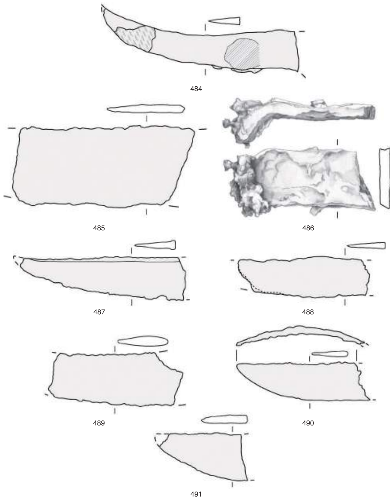
Este, santuario di Reitia. Coltelli di ferro – Eisenmesser: 484–491. Scala 1 : 1.
