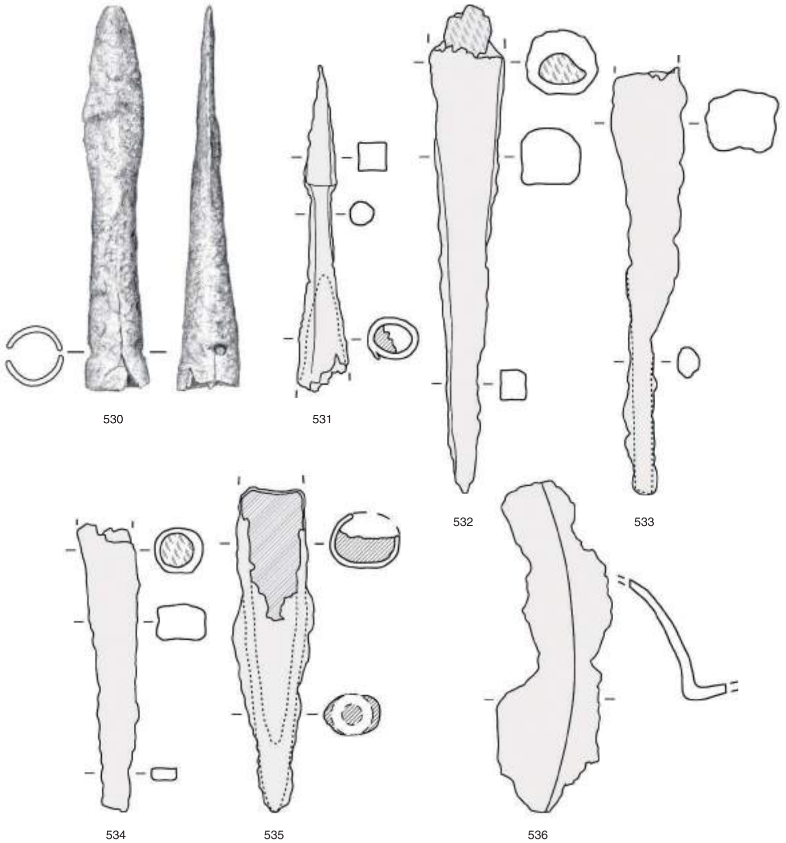
Este, santuario di Reitia. Punta di gavelotto – Speerspitze: 530–531. Tallone di lancia – Lanzenschuh: 532–535. Umbone di scudo – Schildbuckel: 536. Scala 1 : 1.
