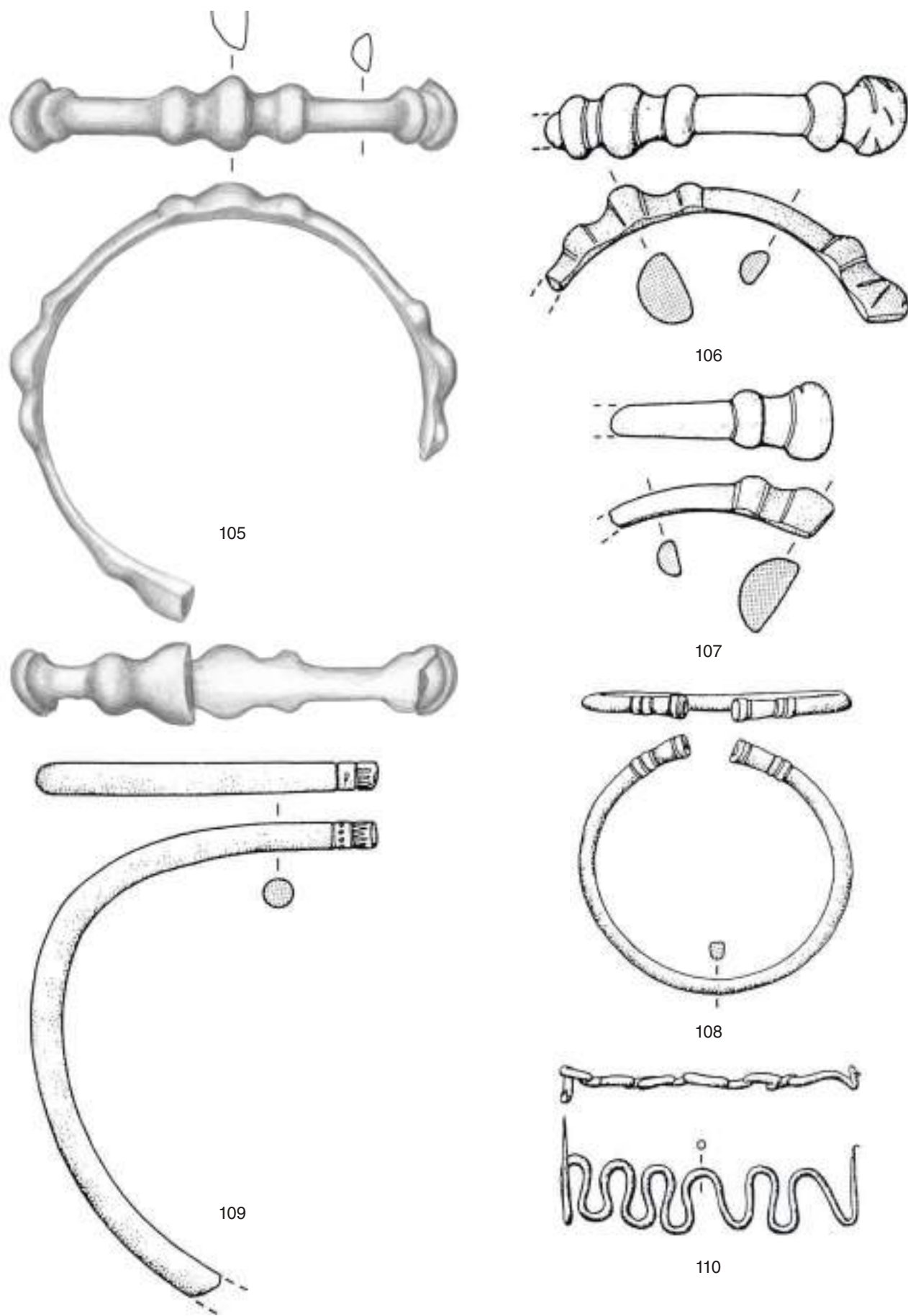
Este, santuario di Reitia. Armille – Armringe: 105–110. Scala 1 : 1.
