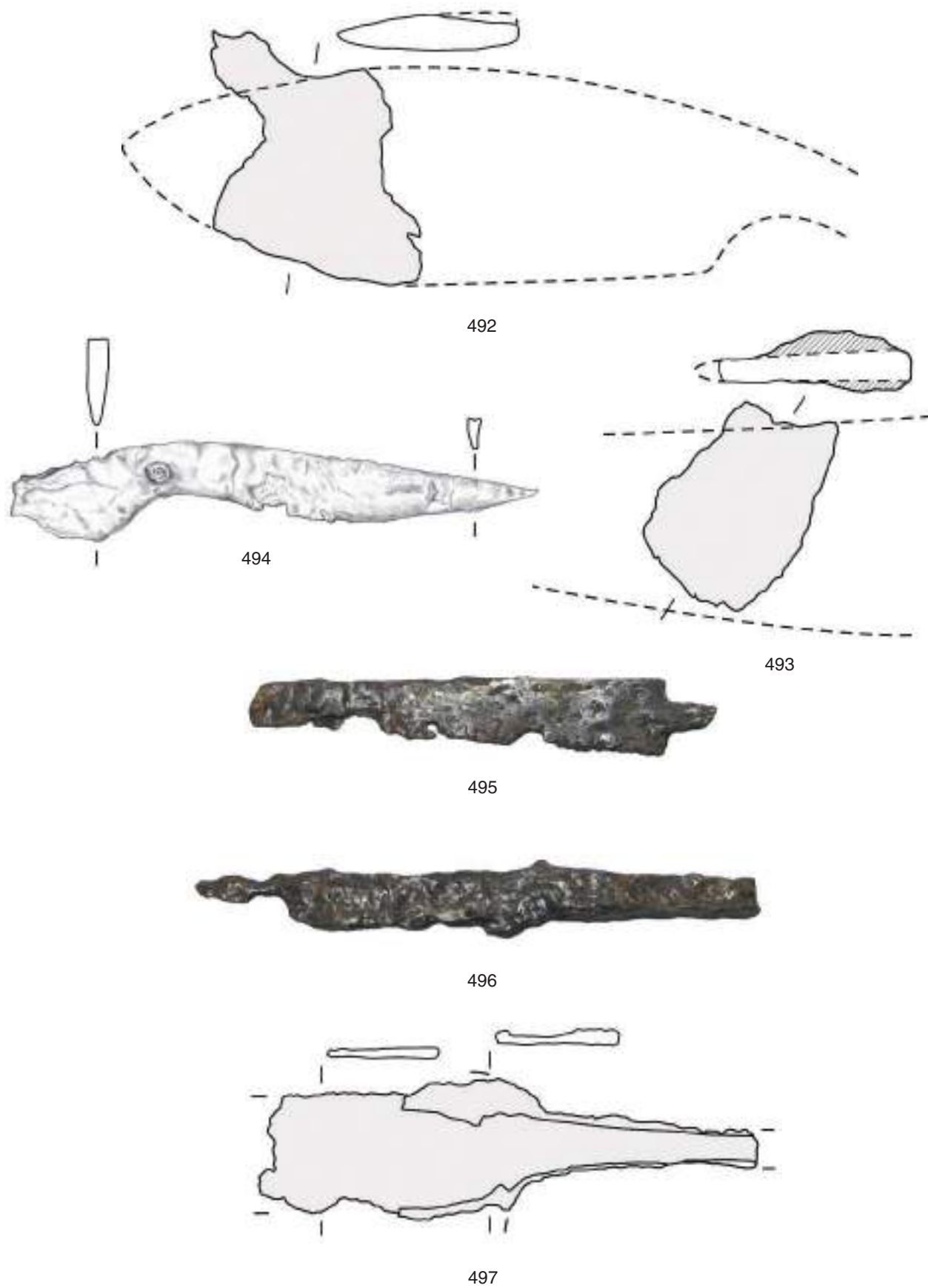
Este, santuario di Reitia. Coltelli di ferro – Eisenmesser: 492–497. Scala 1 : 1.
