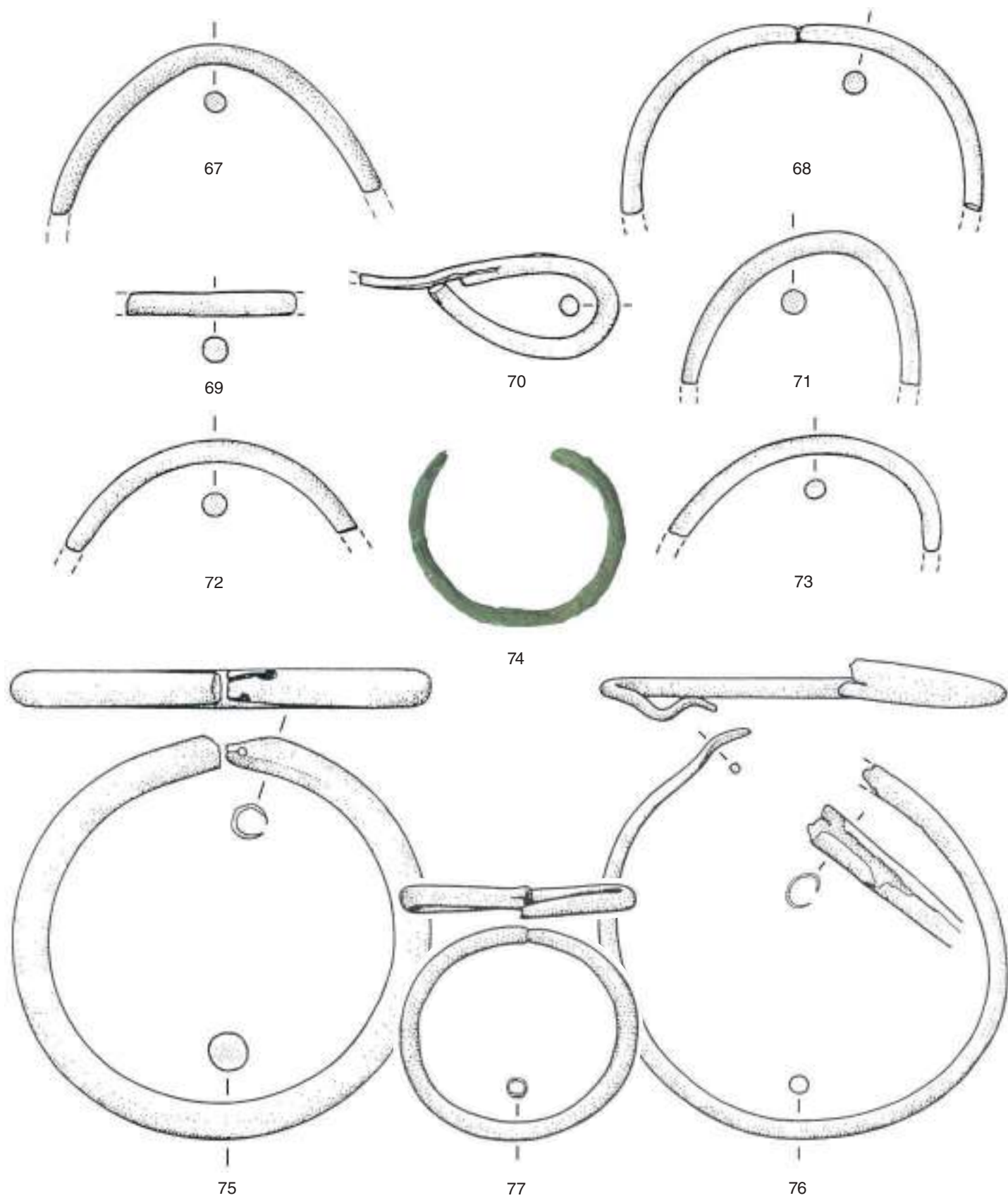
Este, santuario di Reitia. Armille – Armringe: 67-77. Scala 1 : 1.
