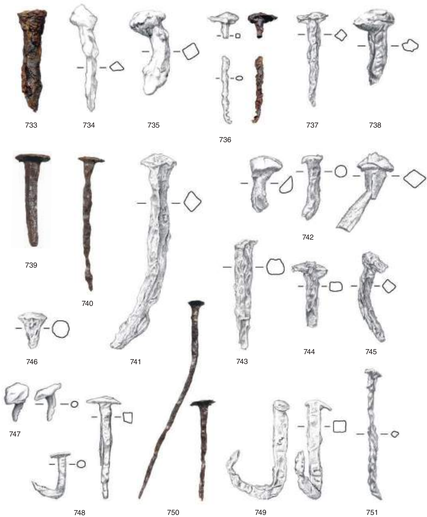
Este, santuario di Reitia. Chiodi di ferro – Eisennägel: 733–751. Scala 1 : 1.
