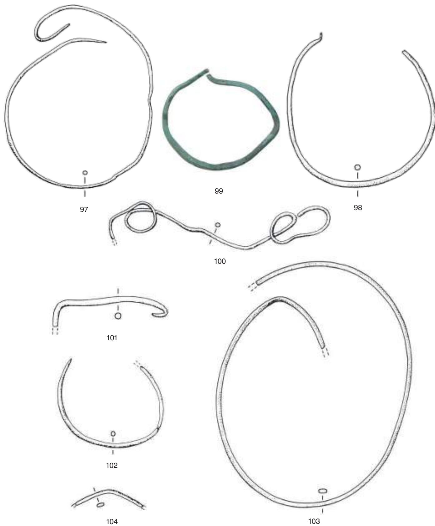
Este, santuario di Reitia. Armille – Armringe: 97–104. Scala 1 : 1.
