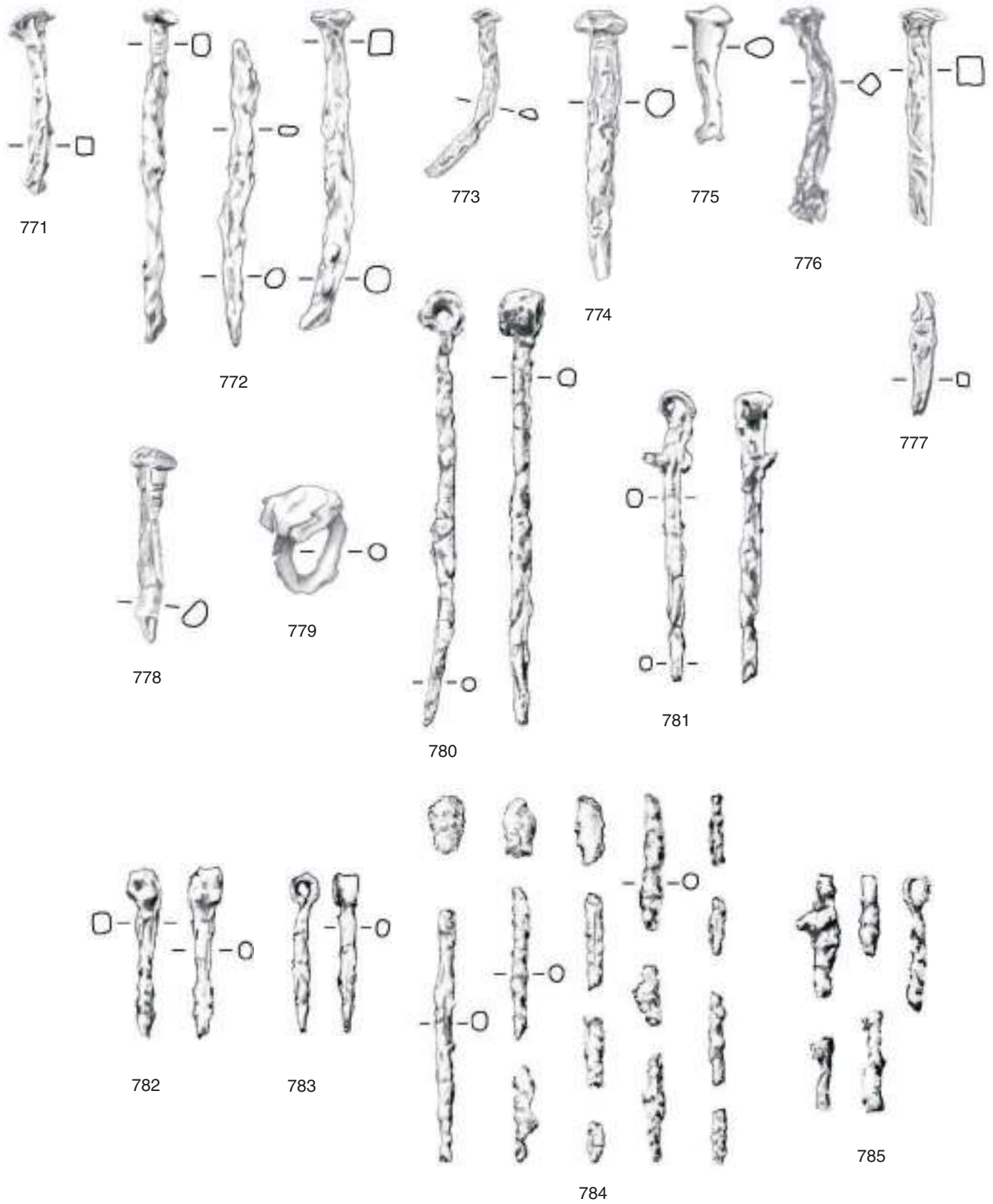
Este, santuario di Reitia. Chiodi di ferro – Eisennägel: 771–785. Scala 1 : 1.
