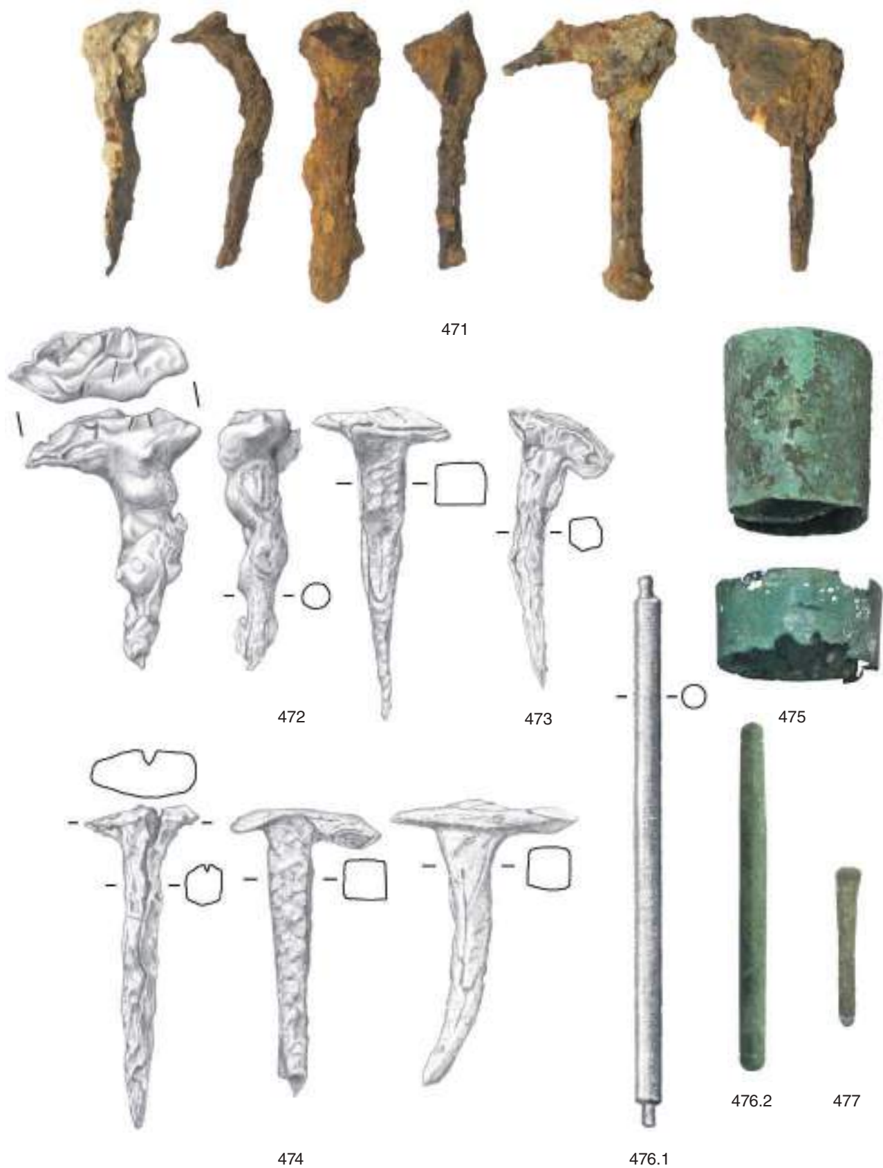
Este, santuario di Reitia. Grappe di ferro – Eisenklammern: 471–474. Minuteria metallica – Metallische Kleinteile: 475–477. Scala 1 : 1.
