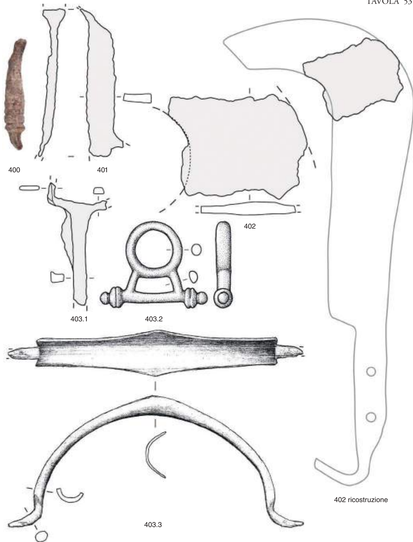
Este, santuario di Reitia. Strumenti – Geräte: 400–403.1 Anello – Ring: 403.2. Presa – Griff: 403.3. Scala 1 : 1. Ricostruzione – Rekonstruktion: 402. Scala 2 : 3.
