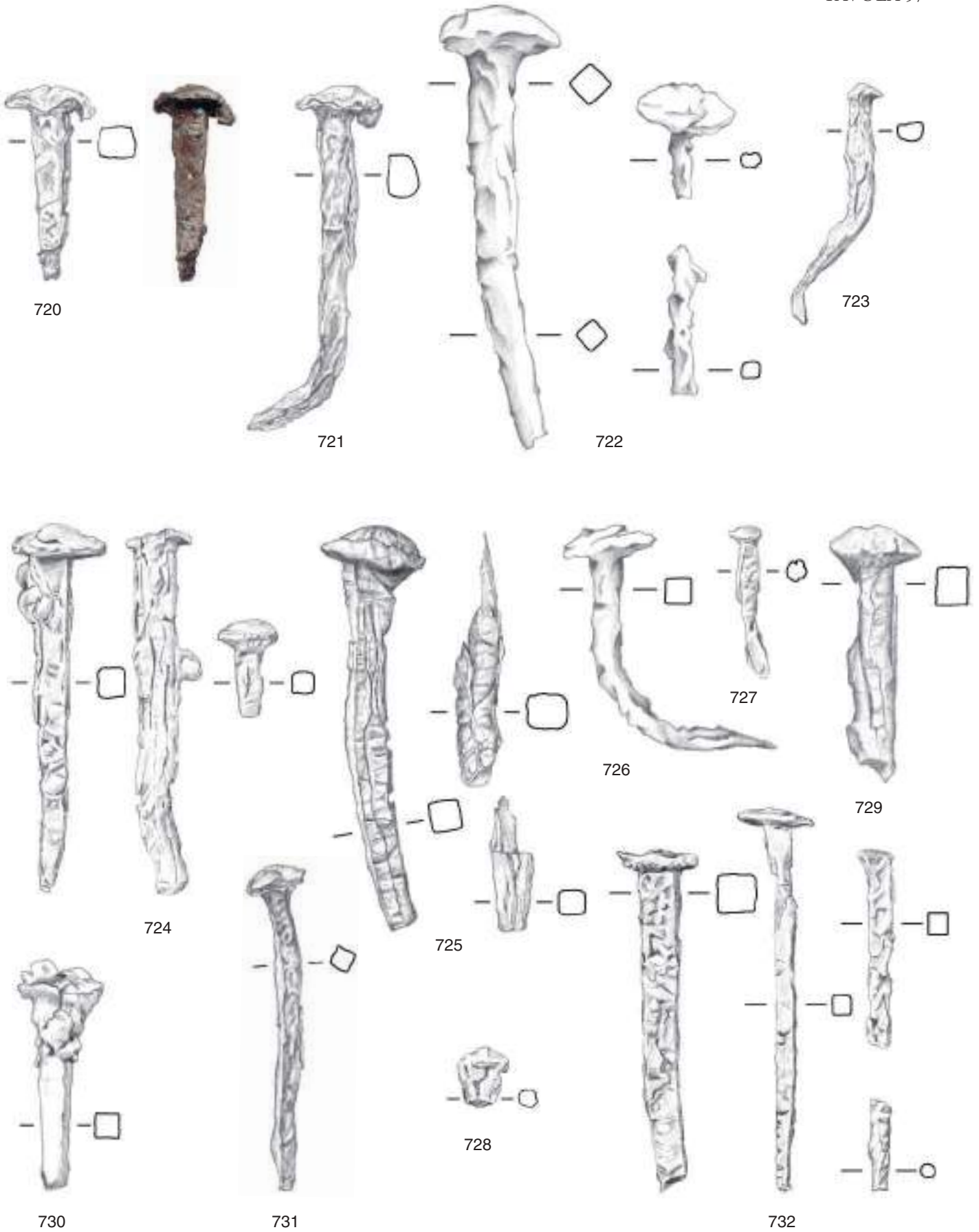
Este, santuario di Reitia. Chiodi di ferro – Eisennägel: 720–732. Scala 1 : 1.
