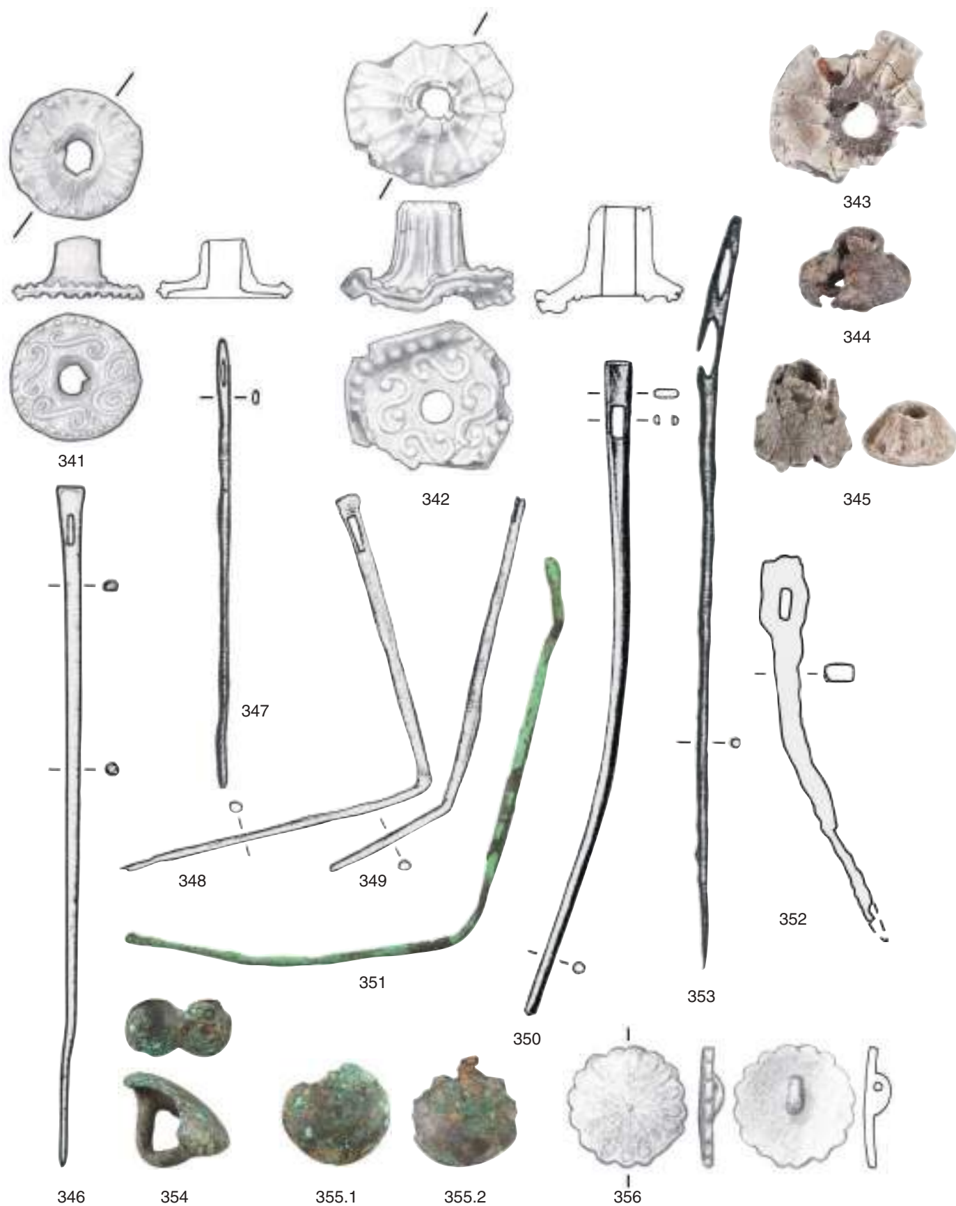
Este, santuario di Reitia. Strumenti da filatura, tessitura e cucito – Instrumente zum Spinnen, Weben und Nähen: 341–345 Piombo – Blei. 346–356 Bronzo – Bronze. Scala 1 : 1.
