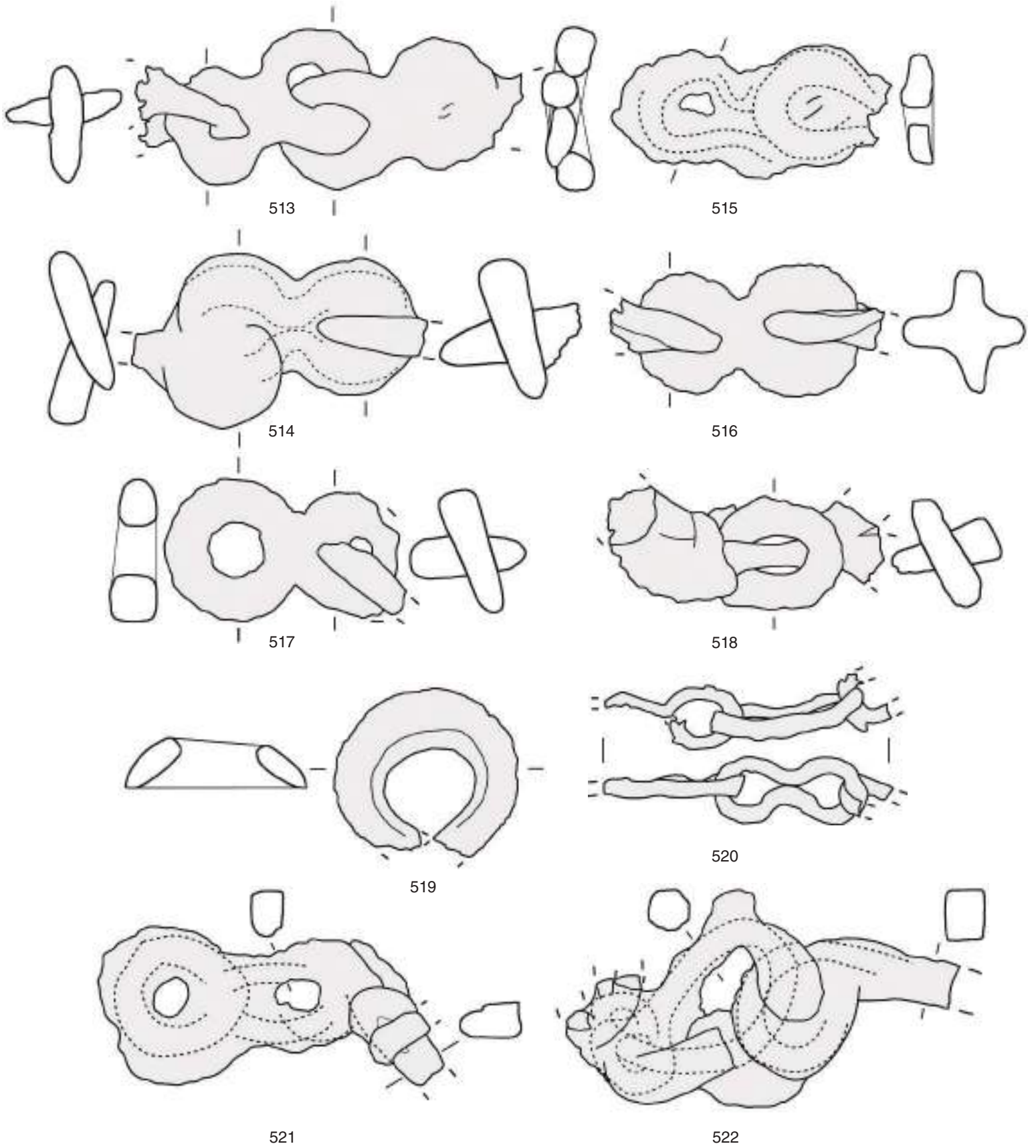
Este, santuario di Reitia. Catene da cintura in ferro – Eiserne Gürtelketten: 513–522. Scala 1 : 1.
