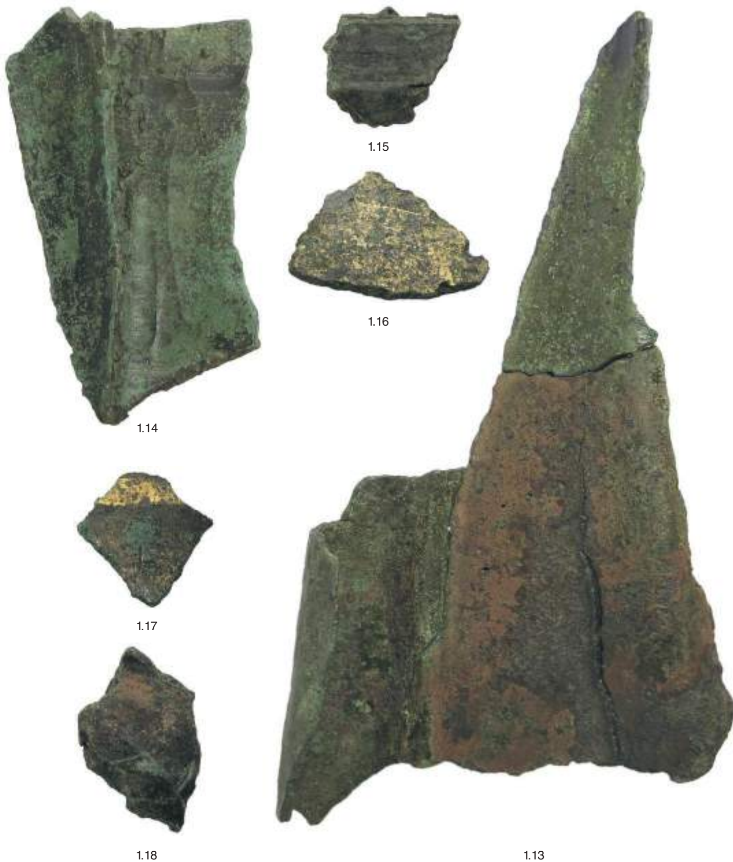
Este, santuario di Reitia. Frammenti di statua di bronzo (lati esterni) – Fragmente einer Bronzestatue (Außenseiten): 1.13–1.18. Scala 1 : 1.
