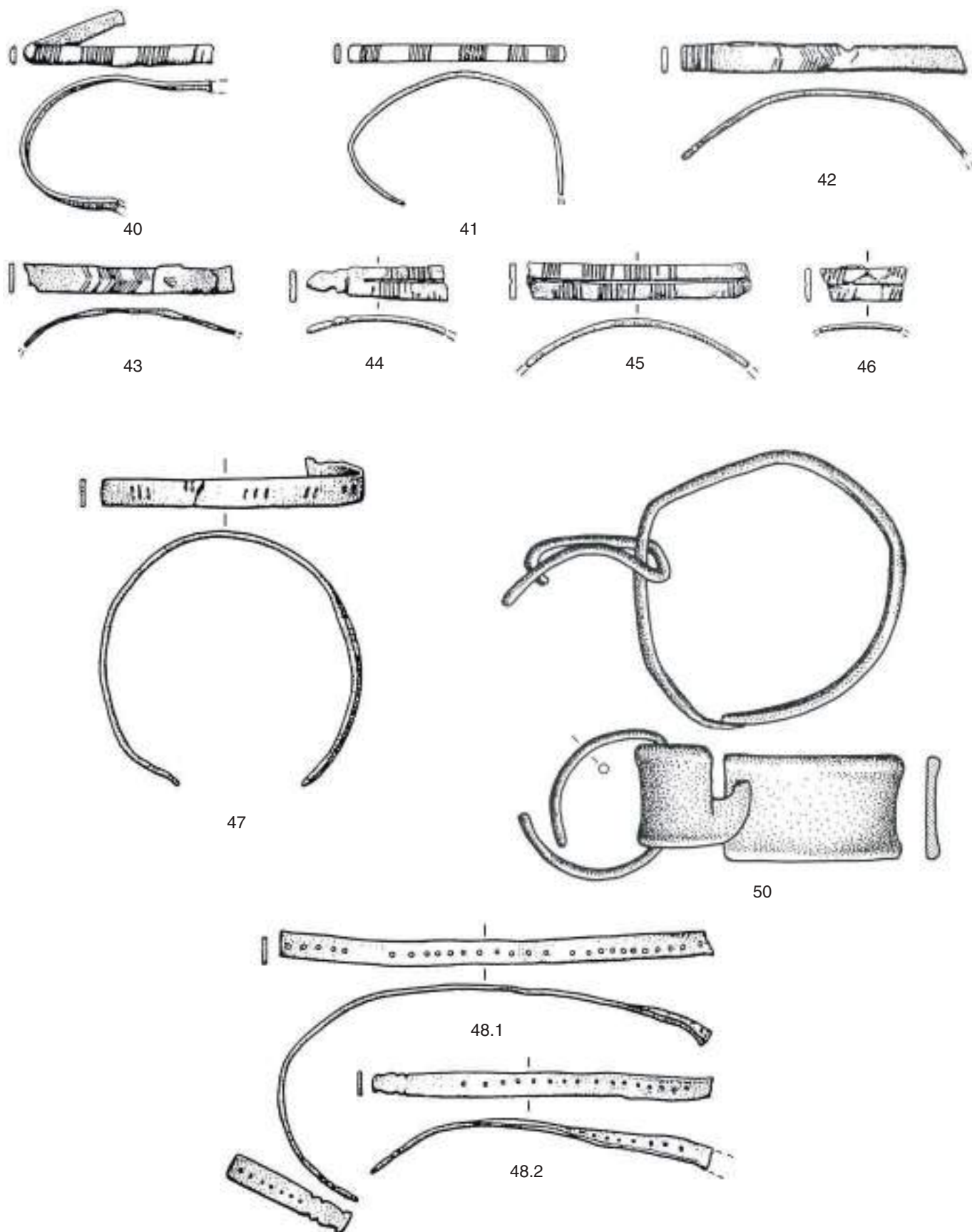
Este, santuario di Reitia. Armille – Armringe: 40–48. 50. Scala 1 : 1.
