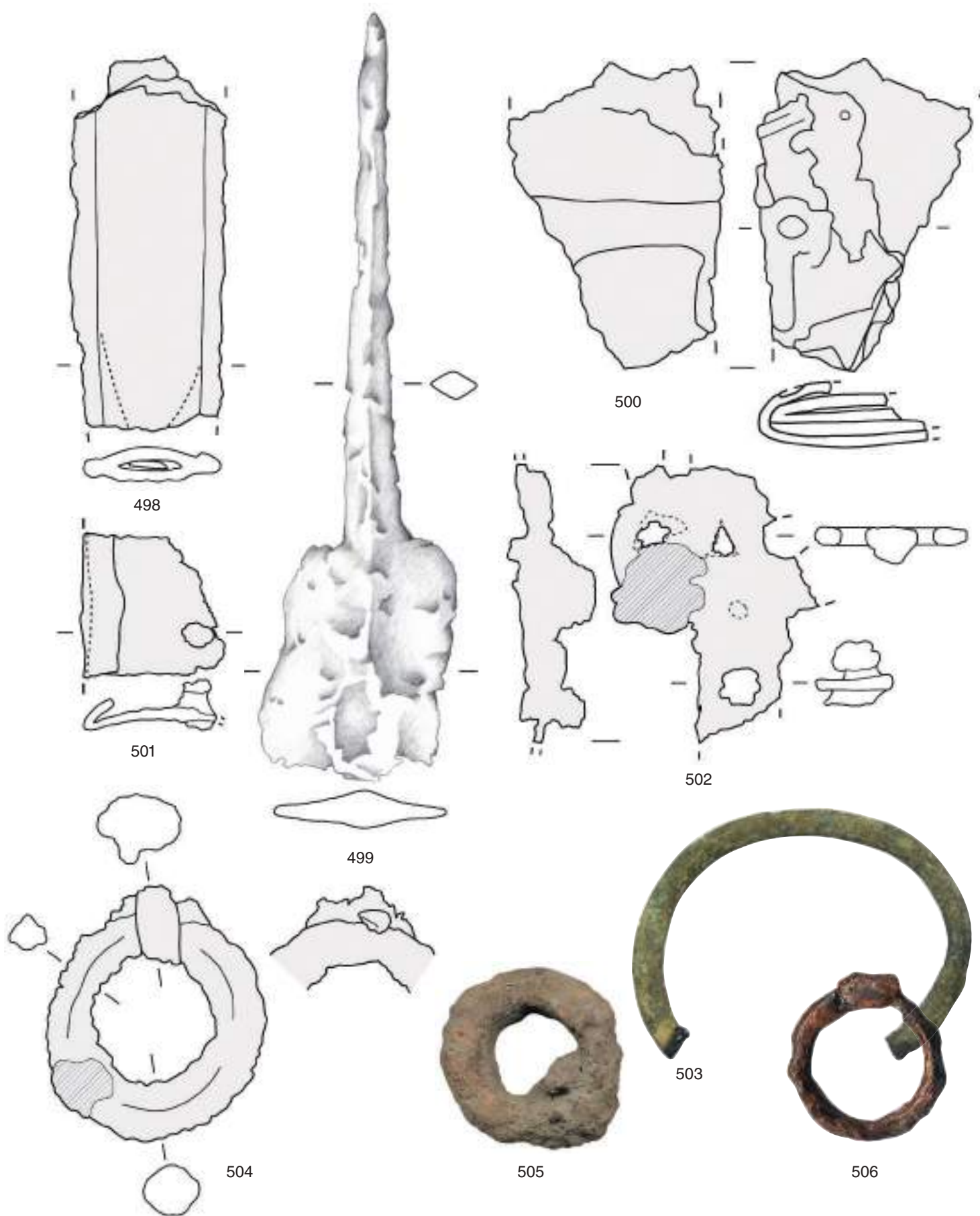
Este, santuario di Reitia. Spada e fodero di spada – Schwert und Schwertscheide: 498–501.
