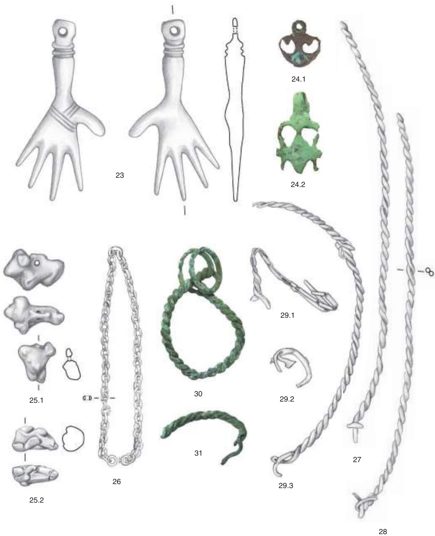
Este, santuario di Reitia. Pendagli – Anhänger: 23–25. Catenella – Kettchen: 26. Torques – Halsringe: 27–31. 23. Scala 2 : 1. 24–31. Scala 1 : 1.
