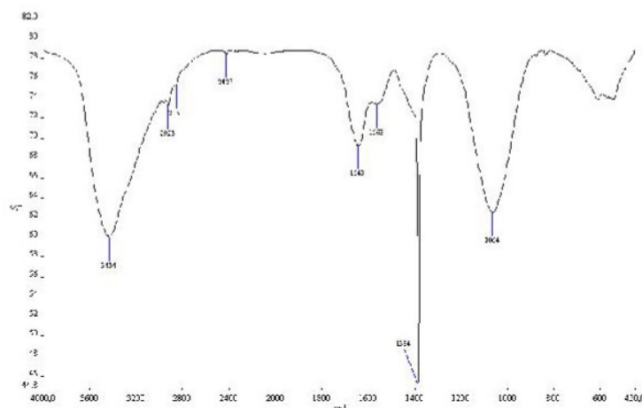
Fig. 1. FT-IR spectrum of Met x -EPS
