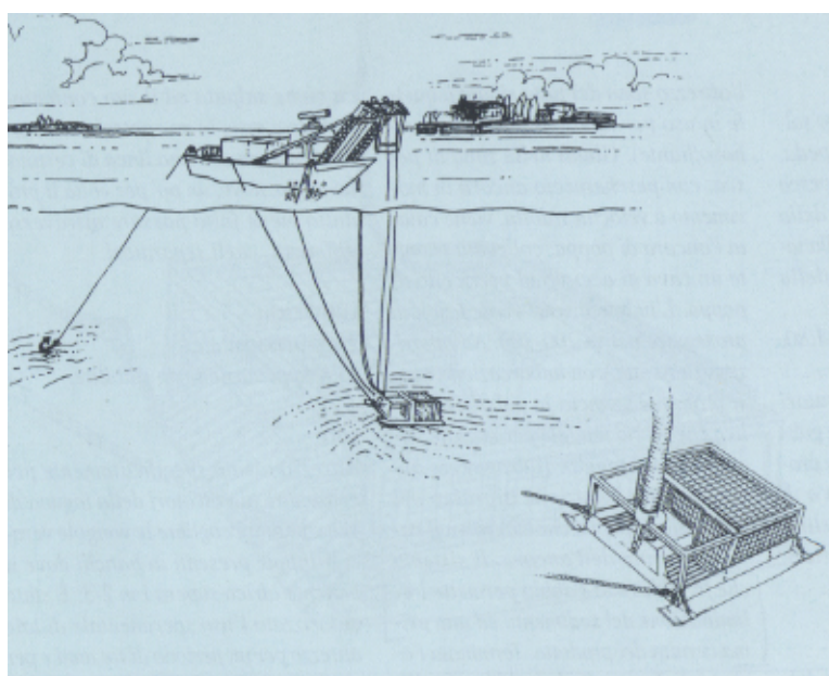
Figure 23. Turbosoffiante
