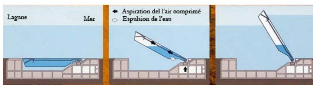
Figure 4. Le fonctionnement des cloisons mobiles du système MOSE (propriété de l'image : Consorzio Venezia Nuova)
