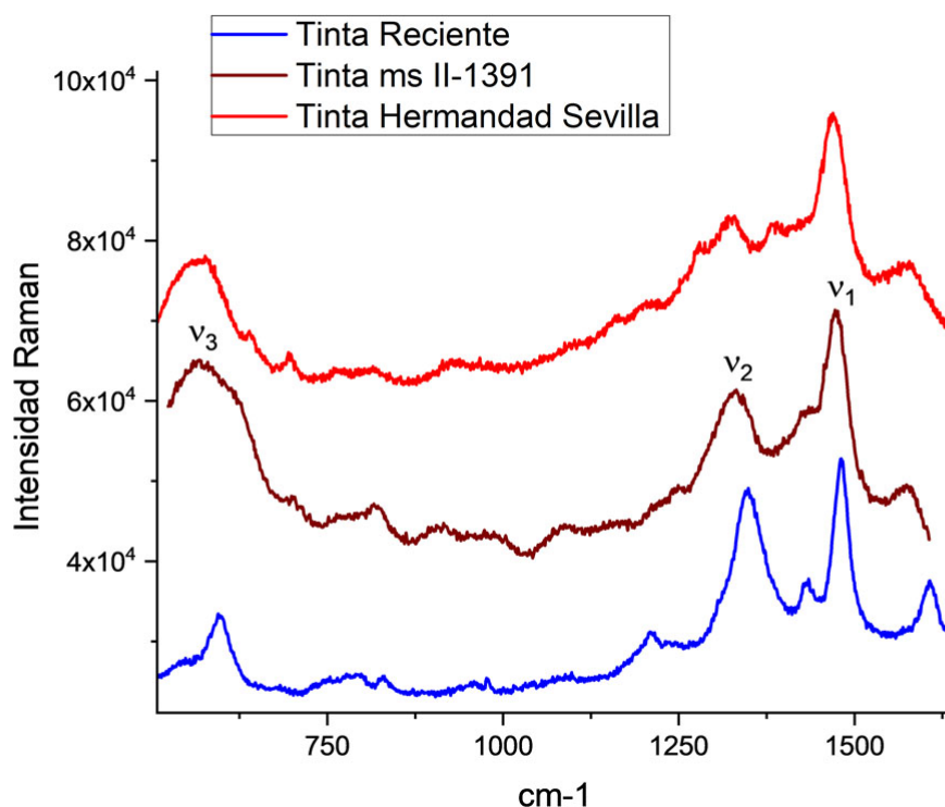
Ilustración 6: Espectros Raman de tinta reciente, preparada en el laboratorio siguiendo la receta Córdoba recogida en Zamorano (2018); espectro Raman más frecuente medido en el manuscrito II/1391 (2); y espectro Raman medido en un manuscrito cedido por la Hermandad de Nuestra Señora del Amparo de Sevilla.
