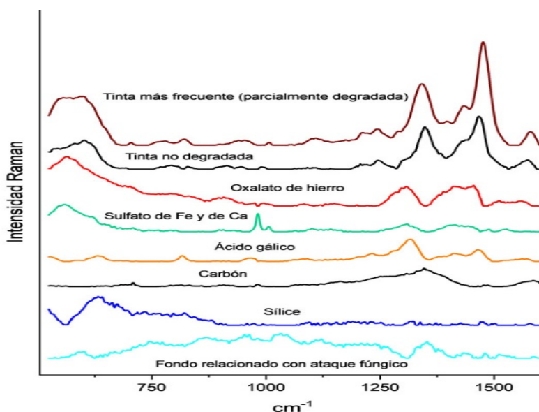
Ilustración 13: Espectros virtuales deducidos mediante el método NMF a partir del análisis de los espectros Raman obtenidos del análisis del manuscrito II/1391 (2)..
