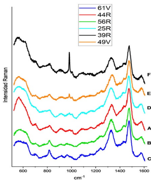
Ilustración 10: Espectros Raman representativos de cada familia de tintas.
