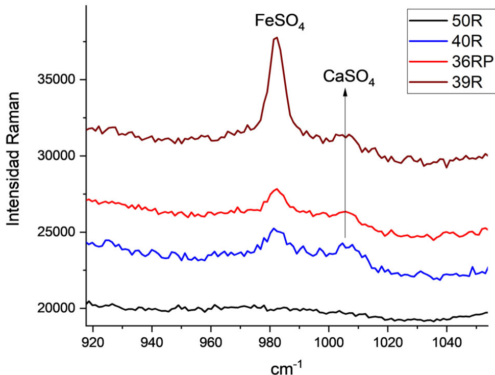
Ilustración 15. Espectros Raman en la región donde aparecen las bandas correspondientes a sulfatos de Fe y de Ca.
