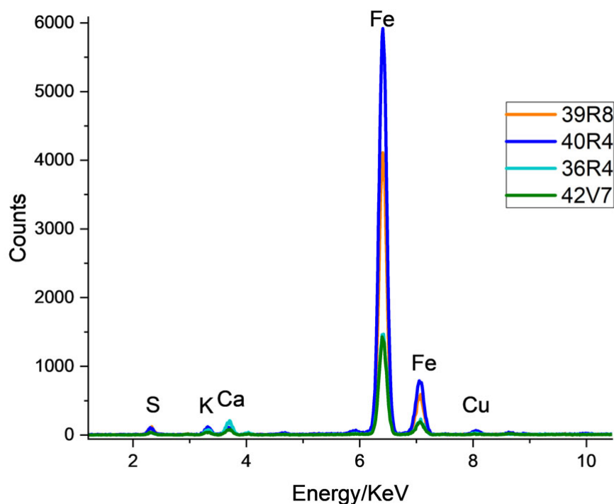
Ilustración 17: Espectros XRF registrados en tintas de los folios indicados en la ilustración correspondientes a los mismos puntos en los que se hicieron los análisis Raman.
