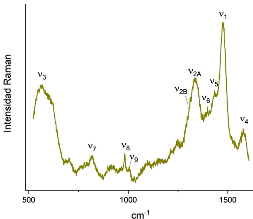
Ilustración 7: Espectro Raman medio en f. 49v del manuscrito con las diferentes bandas y la nomenclatura asignada.
