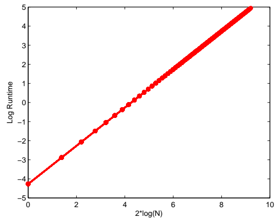
(d) Log Runtime vs 2 \log(N) using QJSU Kernel.
