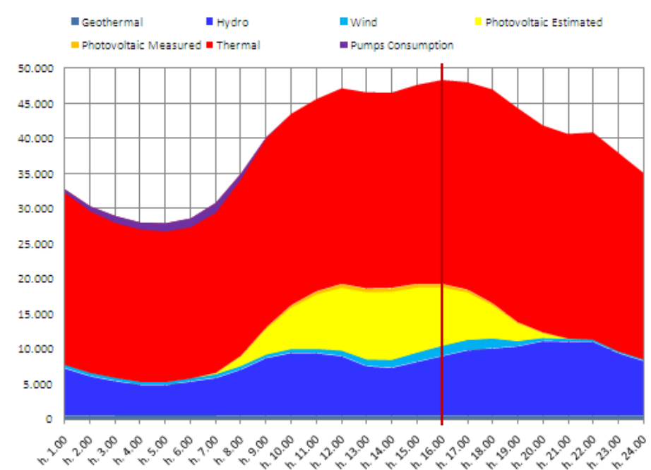
FIG. 12 - PRODUZIONE ELETTRICA DOMESTICA DEL GIORNO 21 LUGLIO IN MW
